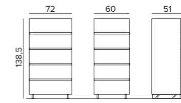
Elemento 5 cassetti
