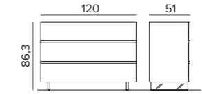
Elemento 3 cassetti
