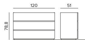
Elemento 3 cassetti P=51 H=78,8
