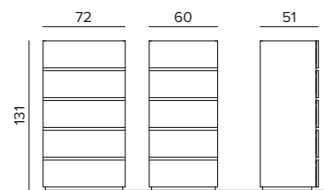
Elemento 5 cassetti P=51 H=131
